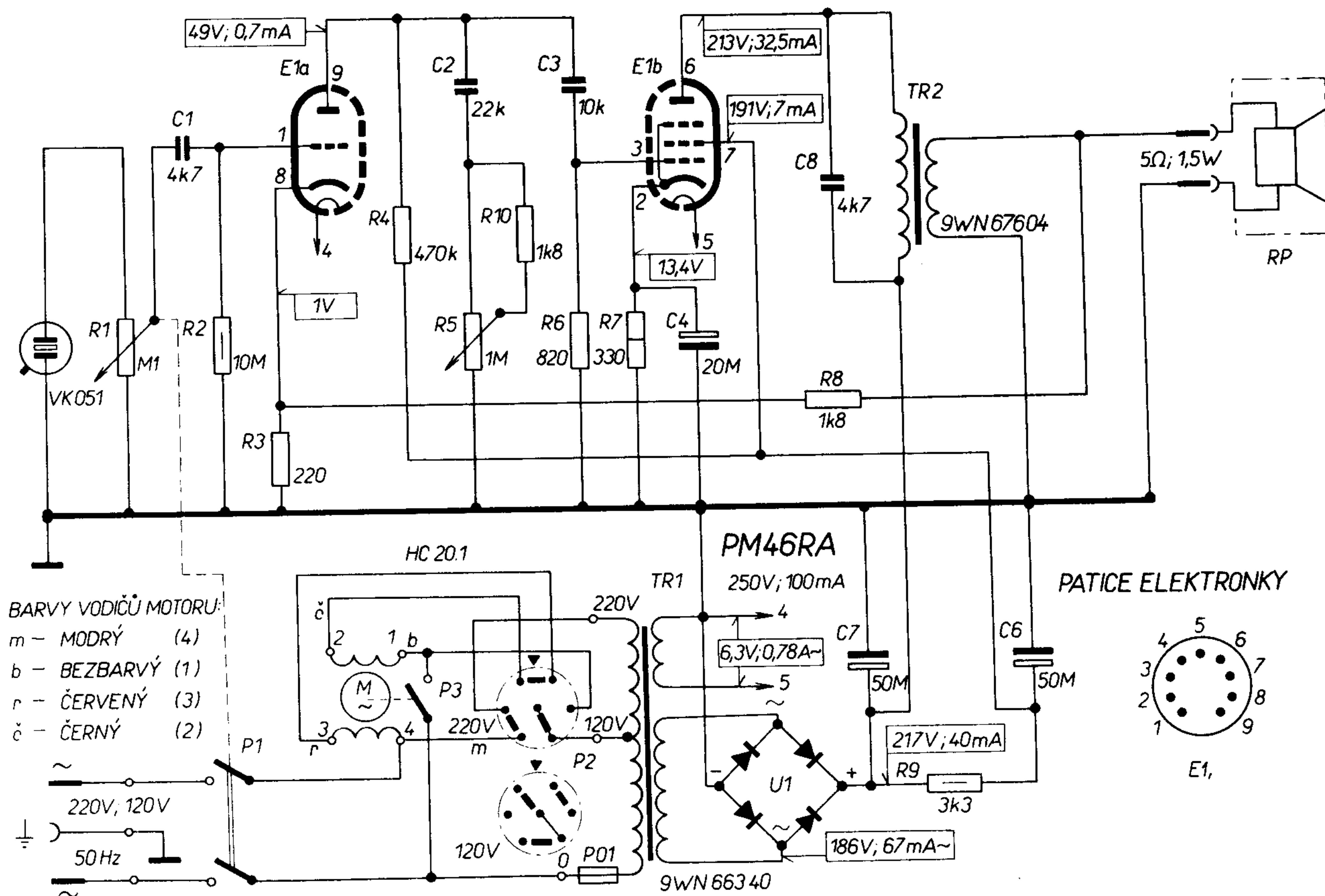
Zapojení nf zesilovače gramofonu GE 080
