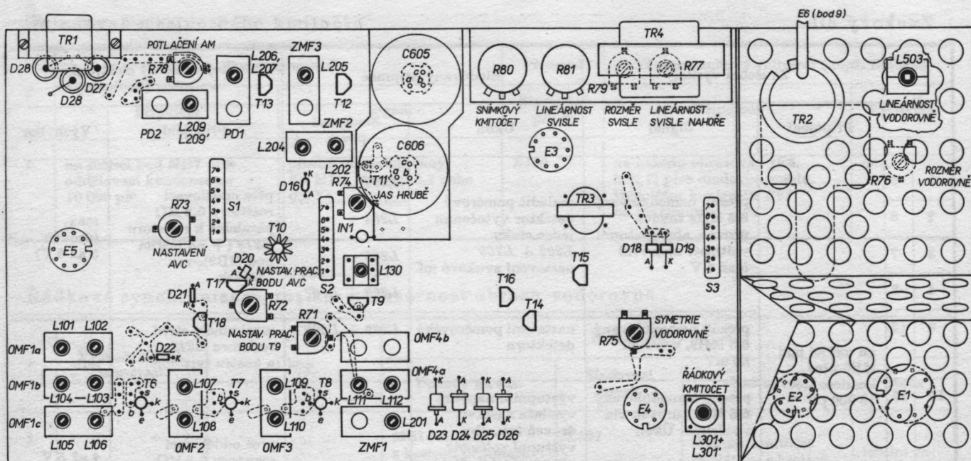
Sladovací prvky na desce s plošnými spoji (za strany součástek)
