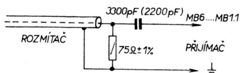
Člen RC pro připojení rozmítače mf
