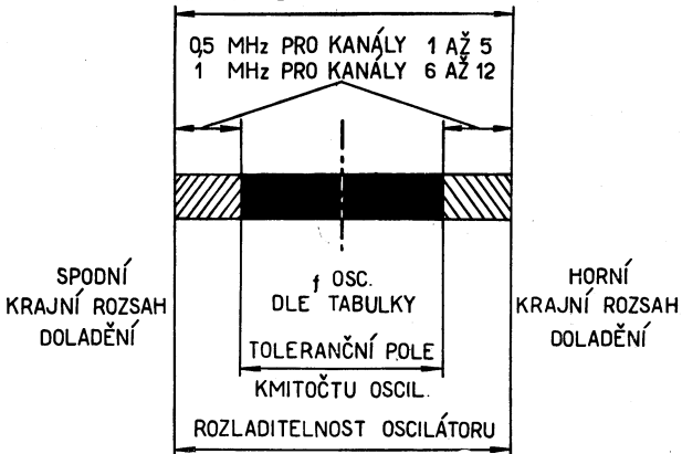
Obr. 1a Toleranční pole kmitočtu oscilátoru
