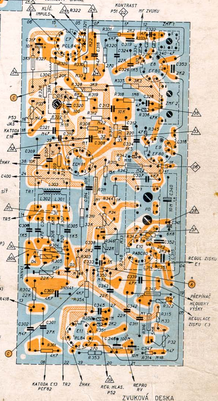
Zapojení televizního přijímače Tesla 4211U-2 „Lotos“, Tesla 4210U-2 „Kamelie“.
