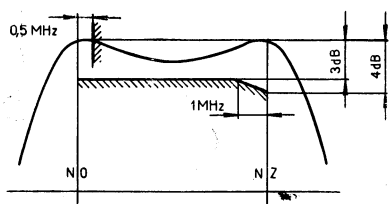
Obr. 1b Kmitočtová charakteristika v části
