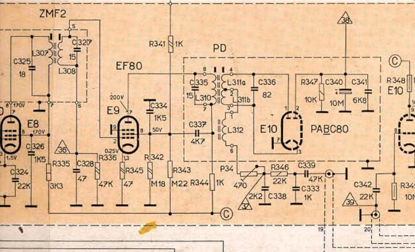
POHLED NA ŠPIČKY MF
