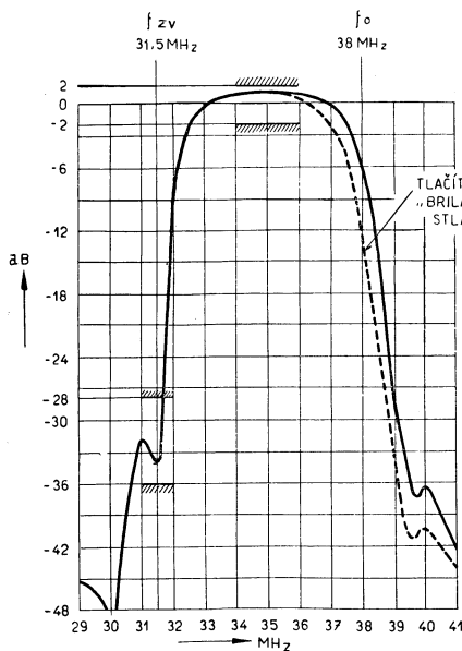
Obr. 5 Kmitočtová charakteristika obrazové mezifrekvence
