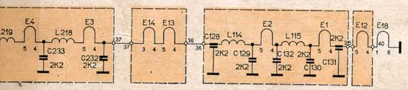
Schéma televizního přijímače Tesla 4211U-2 „Lotos“, Tesla 4210U-2 „Kamelie“.
