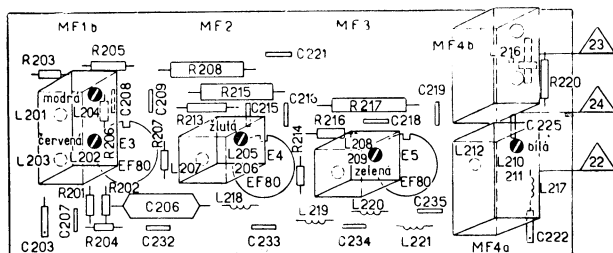
Obr. 4 Deska s plošnými spoji obrazového mezifrekvenčního zesilovače
