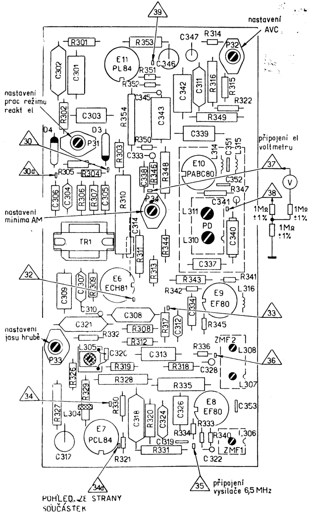
Obr. 7 Deska s plošnými spoji zvukové části přijímače
