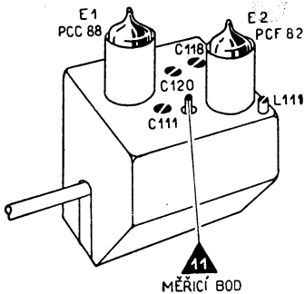
Obr. 2 Nastavovací prvky vř dílu
