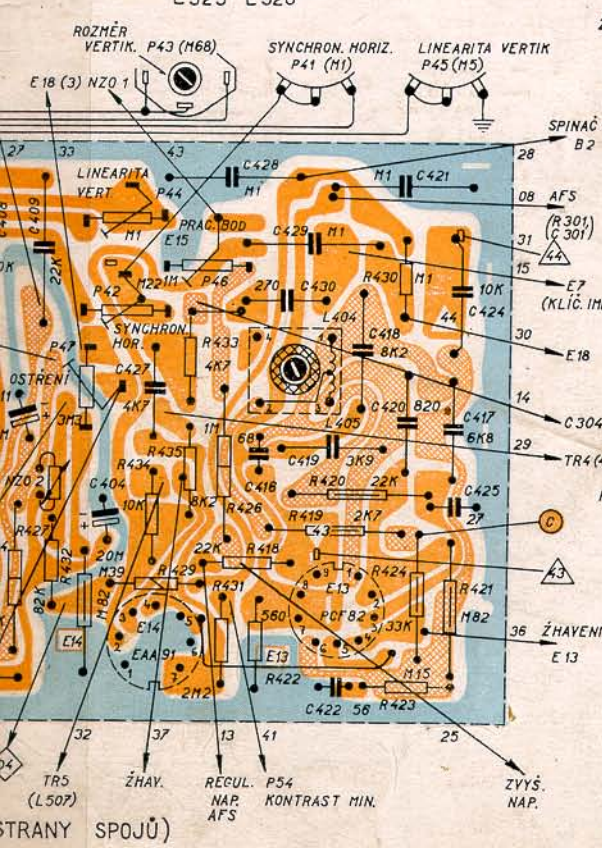
Zapojení televizního přijímače Tesla 4211U-2 „Lotos“, Tesla 4210U-2 „Kamelie“.
