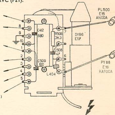
Riadkový transformátor
