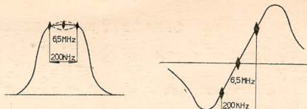
Obr. 14. Frekvenčná charakteristika zvukovej medzifrekvencie
