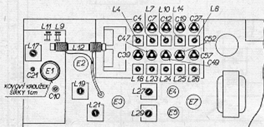
Slaďovací prvky na šasi
