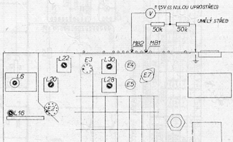
Slaďovací prvky pod šasi
