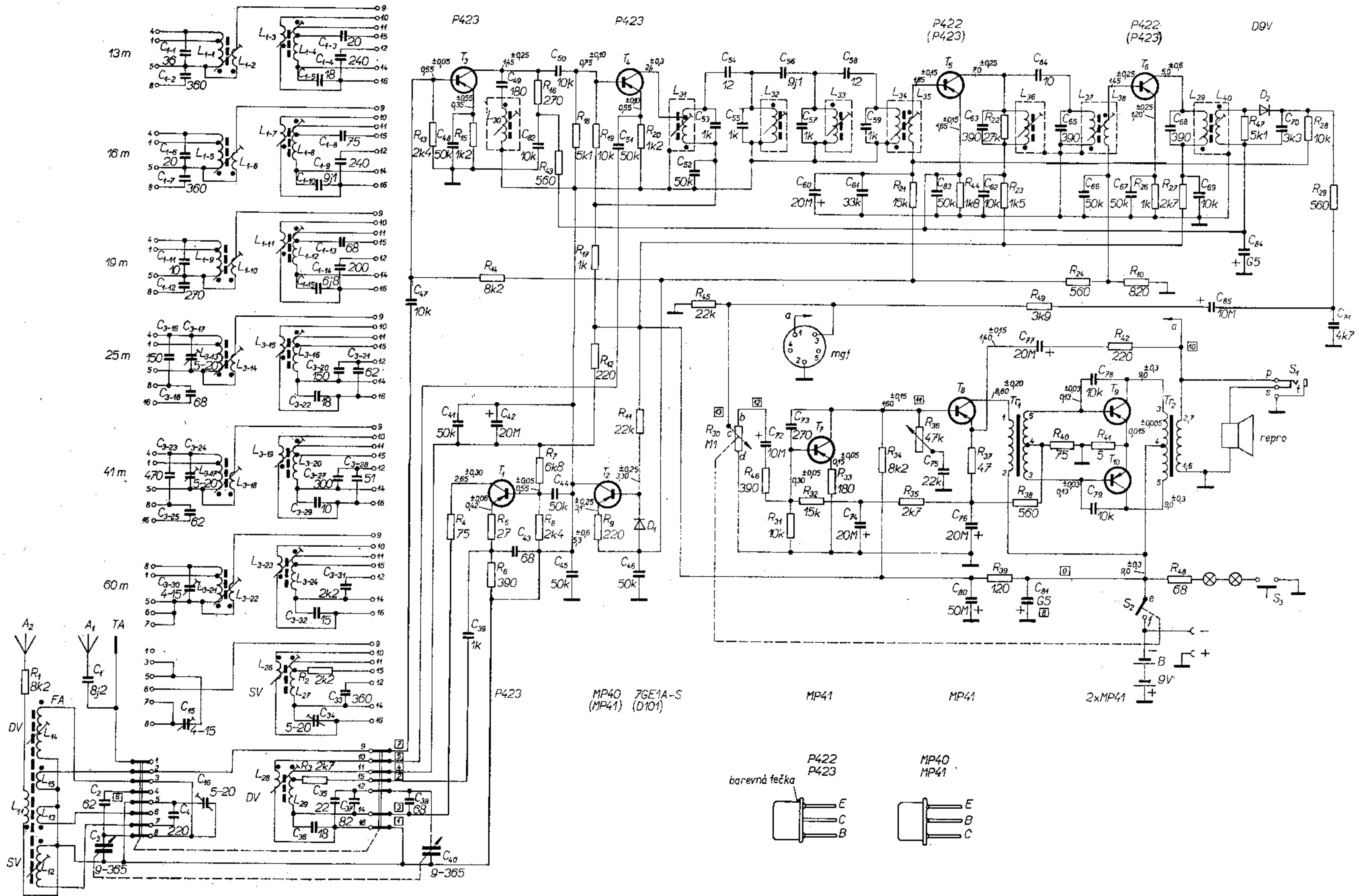
Obr. 1. Schéma přijímače VEF-204
